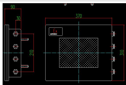
防爆触摸电脑壁挂式示意图
